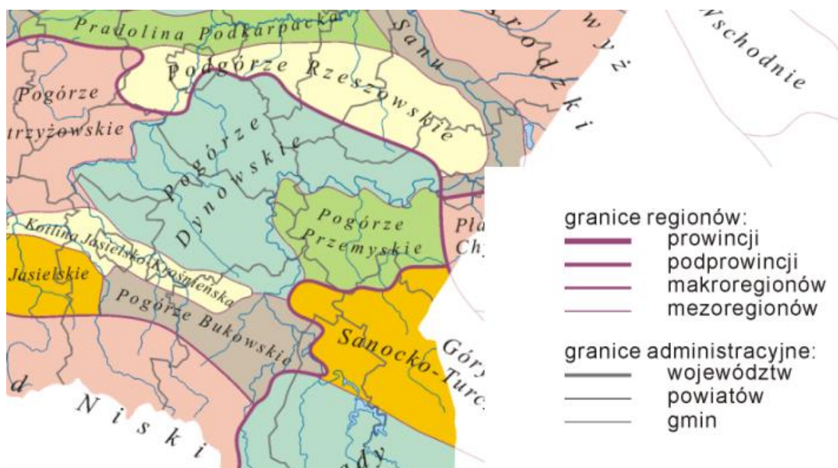
Mapa 6 Położenie fizycznogeograficzne Obszaru Funkcjonalnego „Partnerstwo dla wspólnego rozwoju” według J. Kondrackiego
